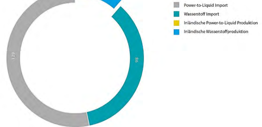
Wasserstoff und Power-to-Liquid Versorgung in NRW im Jahr 2050 in TWh/a
