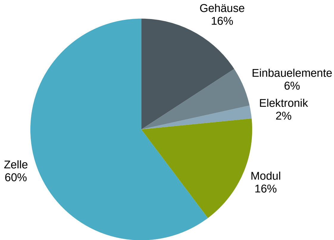
Gewichtsanteile Batteriesystem
